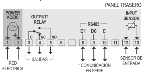
Figura 1 – Conexiones eléctricas
